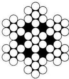
7 x 7 (6 x 7 WSC)
